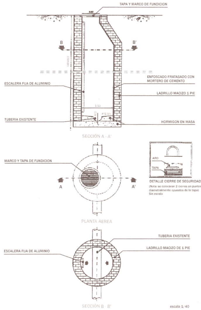
ANEXO IV Modelos y dimensiones de arquetas
